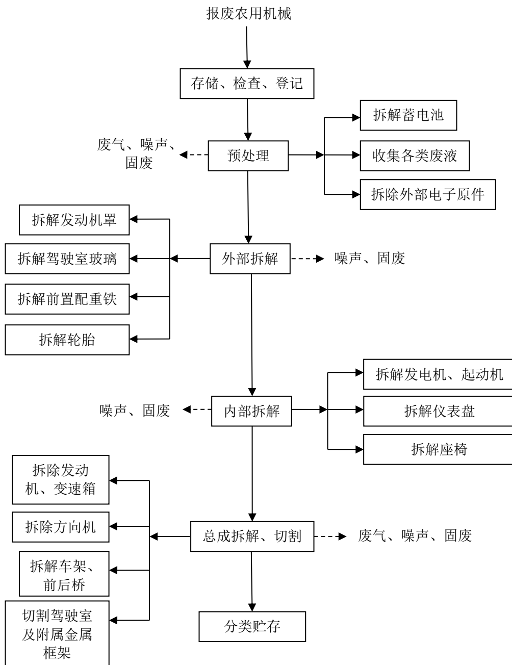
图 2-3 本项目工艺流程图及产污环节图
