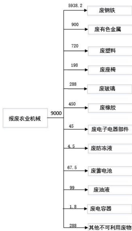
图 2-1 物料平衡图 (单位: t/a)
