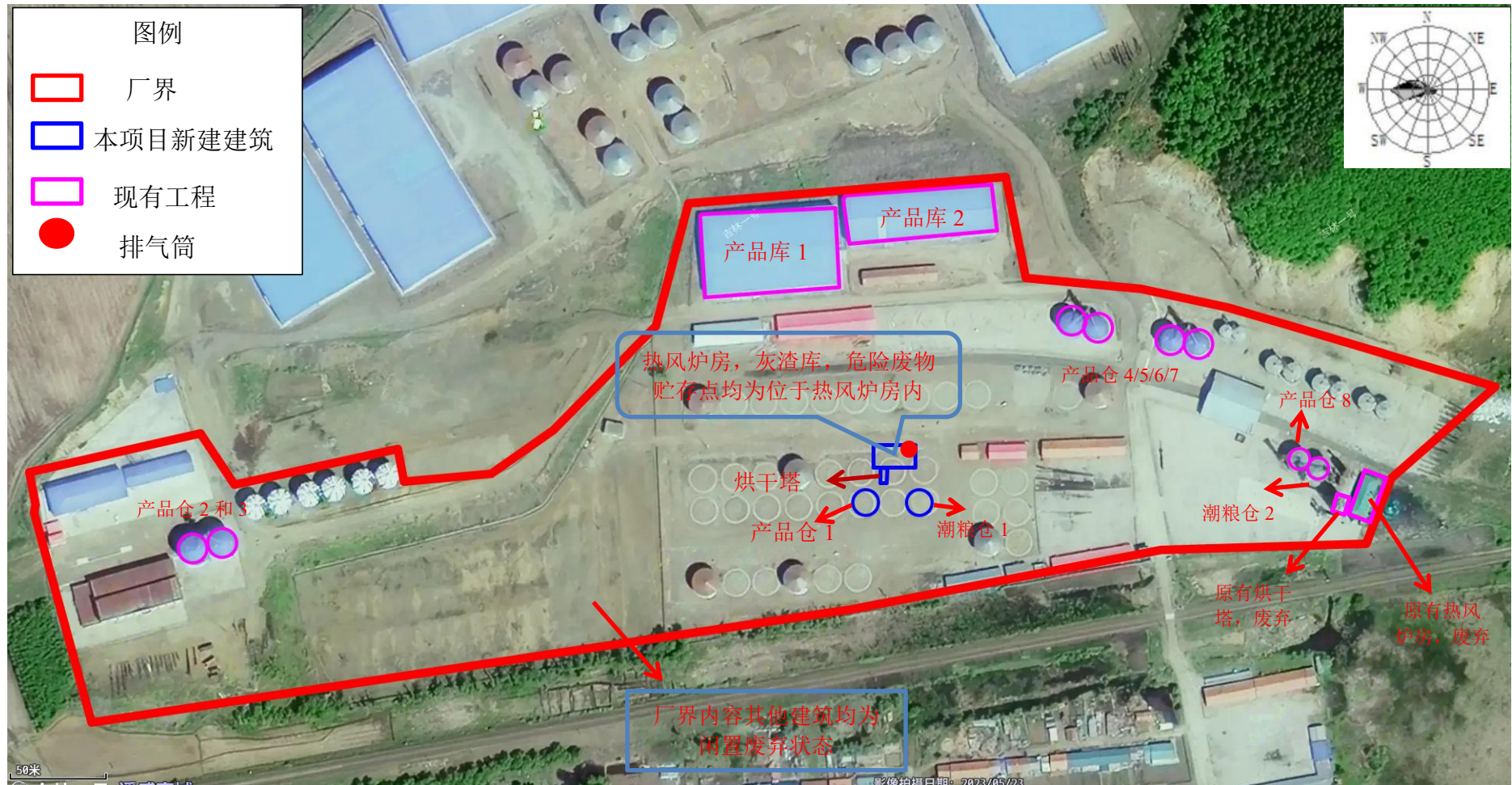
附图 2：本项目范围平面布置图
