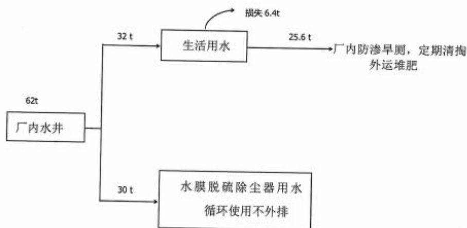
图 2-2 原有工程水量平衡图 (单位: t/a)
